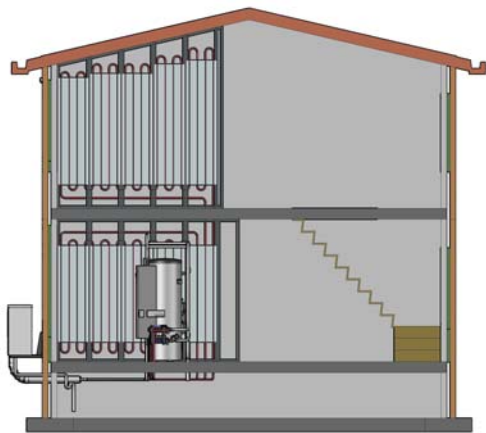
Woning doorsnede linker aanzicht
